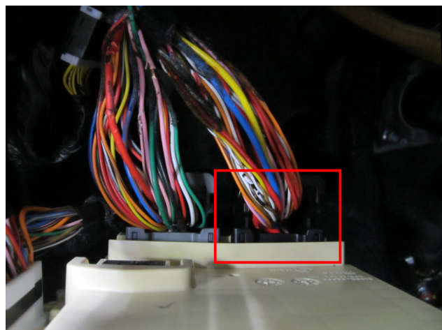
Рис.7 Место подключения к силовым цепям запуска двигателя -2
