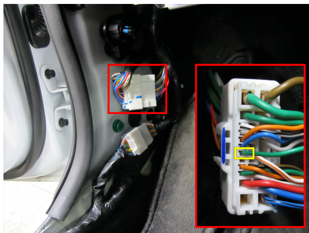
Рис.2 Место подключения (зеленый провод)
