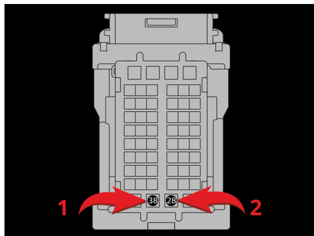
Рис.8 Подключение к силовым цепям запуска двигателя
