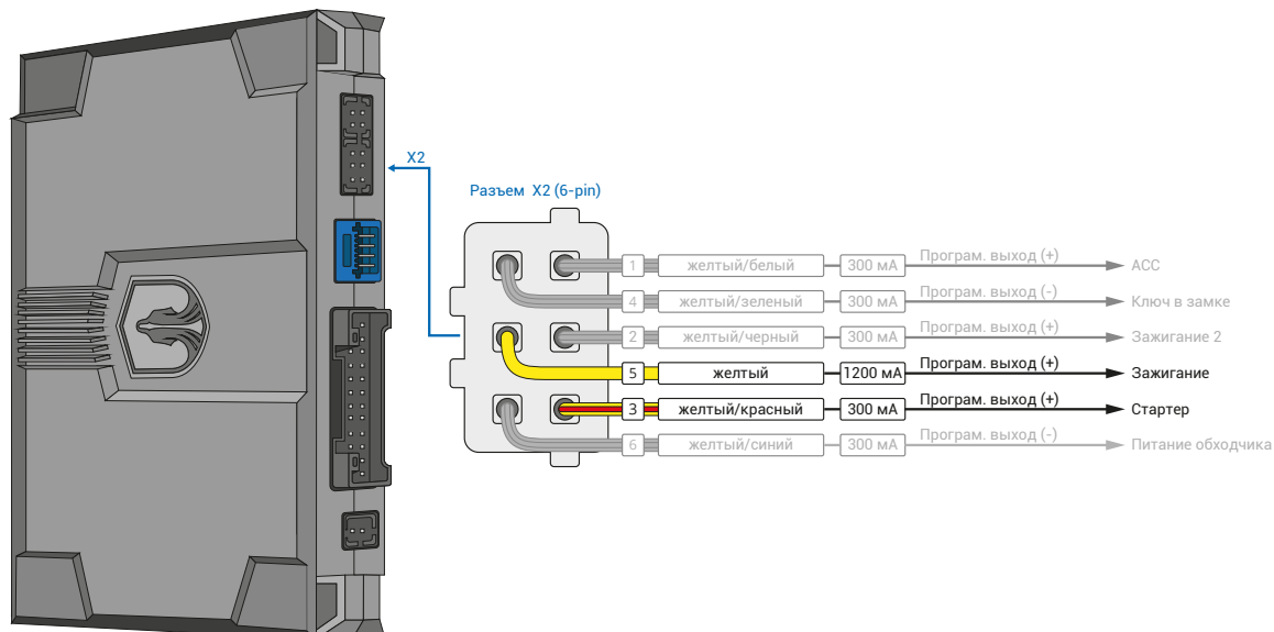
Рис.4 Подключение выходов автозапуска
