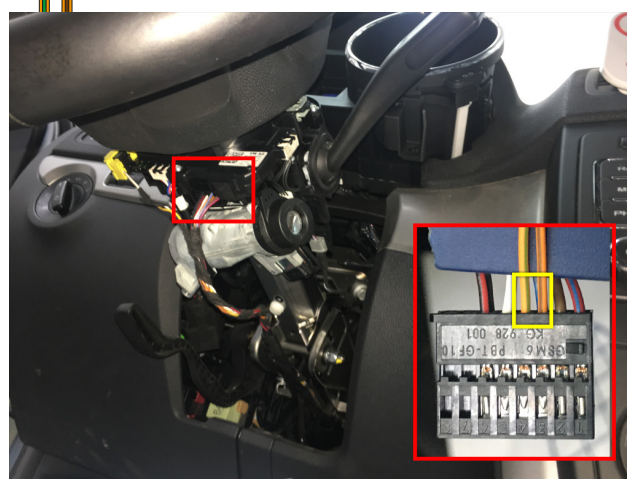
Рис.3 Подключение CAN1
