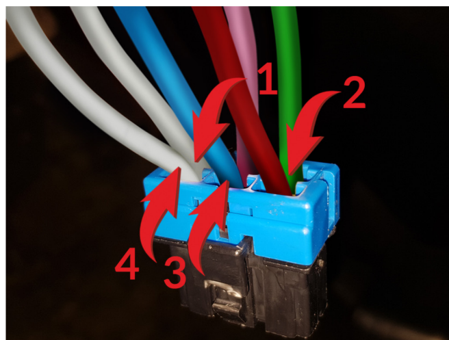
Подключения к силовым цепям запуска двигателя: 1 - АСС (белый провод); 2 - Зажигание 1 (зеленый провод); 3 - Зажигание 2 (синий провод); 4 - Стартер (белый провод).
