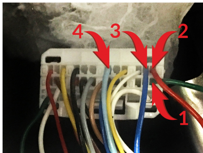
Подключение к силовым цепям замка зажигания 1 – АСС (зеленый провод); 2 – Зажигание 1 (красный провод); 3 – Зажигание 2 (синий провод); 4 – Стартер (голубой провод).
