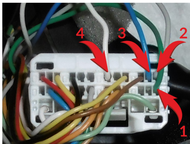
Подключение к силовым цепям замка зажигания 1 - АСС (зеленый провод); 2 - Зажигание 1 (серый провод); 3 - Зажигание 2 (синий провод); 4 - Стартер (белый провод).
