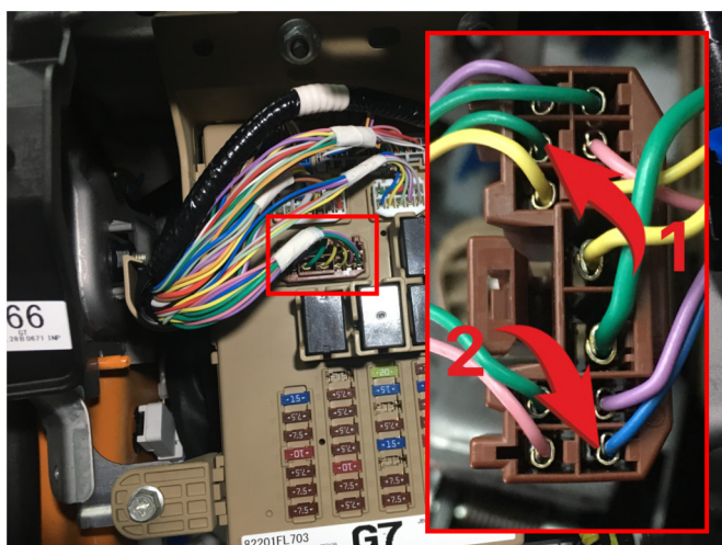
Подключение к силовым цепям 1 - АСС (зеленый провод) 2 - Зажигание (синий провод)
