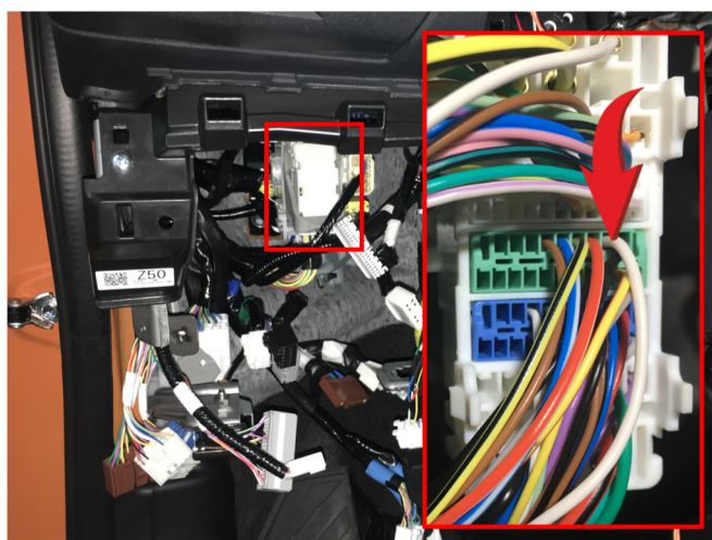
Подключение Стартера (белый провод)
