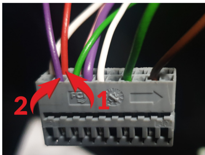
Подключение к цепям запуска двигателя: 1 – Зажигание 1 «+» (красный провод, контакт №32); 2 – Стартер «+» (фиолетовый провод, контакт №22).
