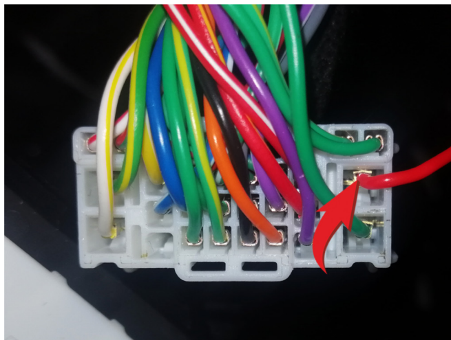
Зажигание 1 (красный провод, контакт № 5)
