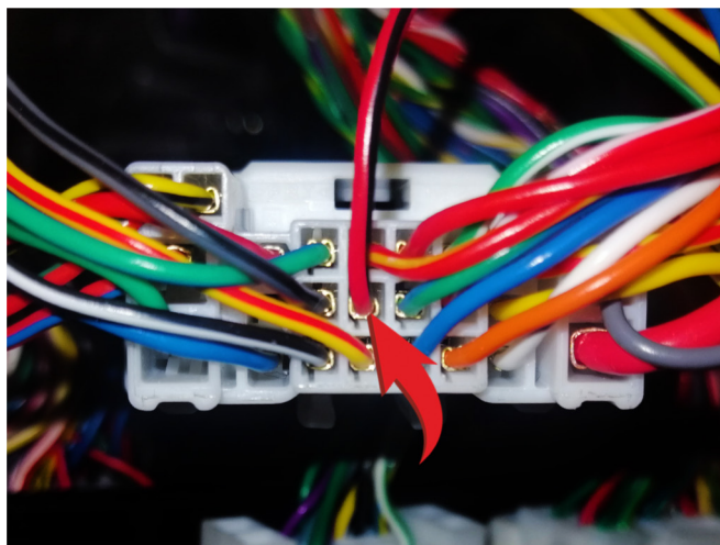
Стартер (красный/черный провод, контакт № 15)
