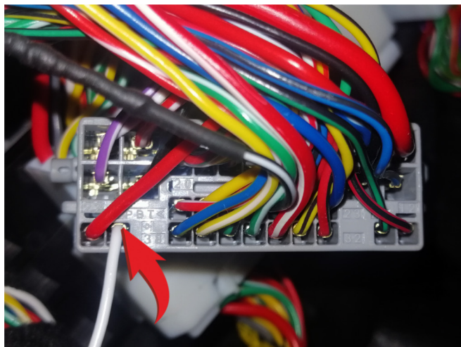
ACC (белый провод, контакт № 39)
