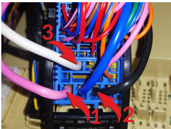
Подключение к цепям запуска двигателя: 1 - Зажигание 1 (розовый провод); 2 - Зажигание 2 (черный провод); 3 - Стартер (белый провод)
