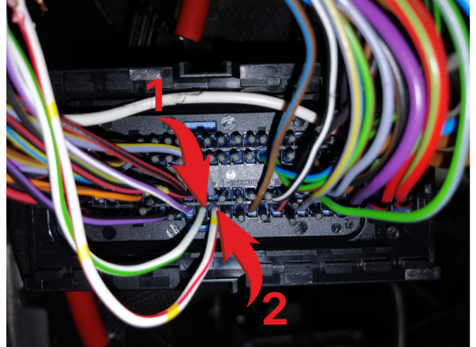
Подключение стартера: 1 - Стартер «-» (белый/зеленый провод); 2 - Стартер «-» (белый/красный провод)
