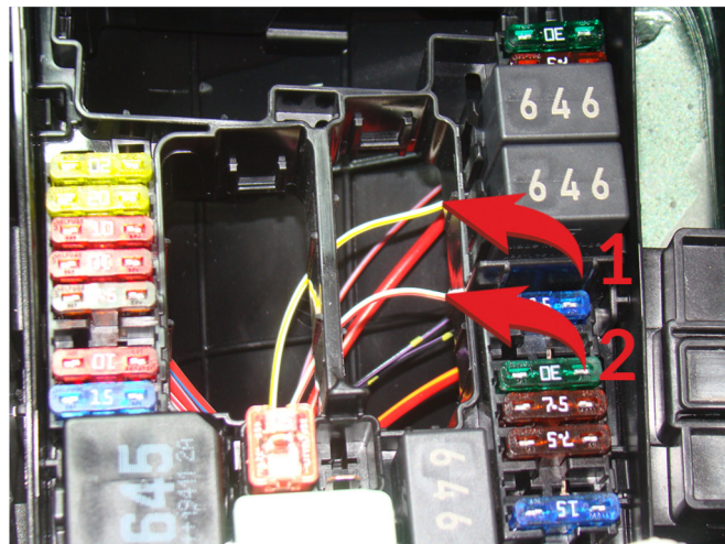
Подключение стартера:
