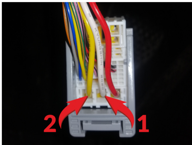
1 – Зажигание 1 (белый провод, контакт № 26); 2 – Зажигание 2 (желтый провод, контакт № 17)
