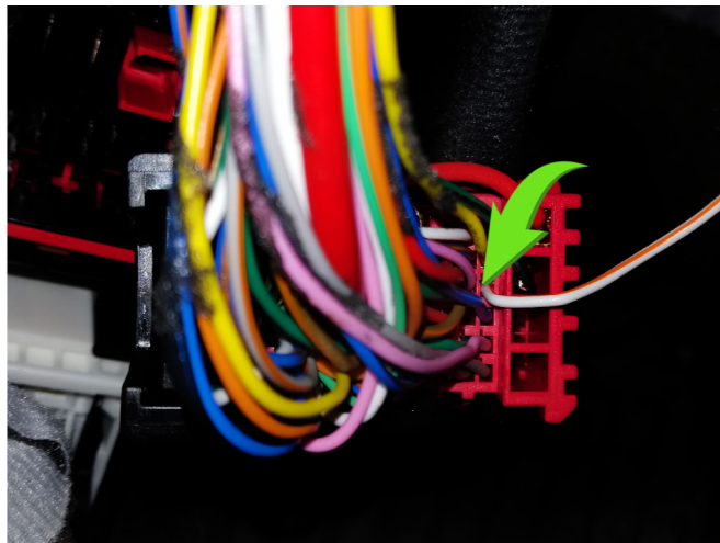
Шина данных (белый/оранжевый провод, контакт № 25)
