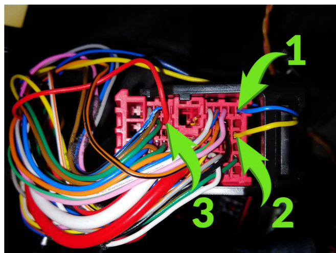
Подключение к цепям запуска двигателя: 1 – Зажигание 1 (синий/черный провод, контакт № 42); 2 – Зажигание 2 (желтый провод, контакт № 26); 3 – Стартер (красный провод, контакт № 39).
