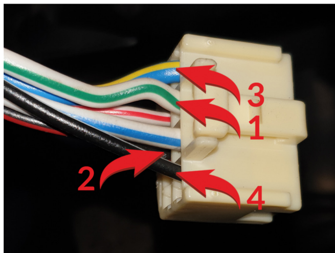
Подключение к цепям запуска: 1 - АСС (белый/зеленый провод); 2 - Зажигание 1 (черный/красный провод); 3 - Зажигание 2 (синий/желтый провод); 4 - Стартер (черный/юедый провод).
