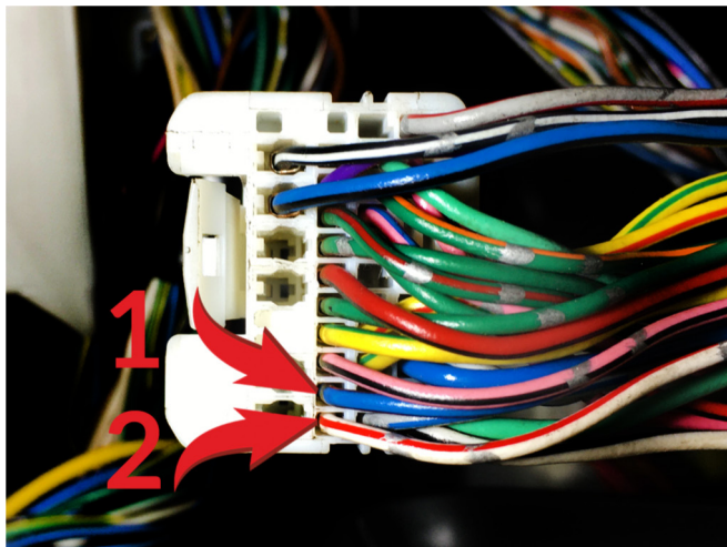
Подключение IMO, IMI: 1 - IMO (синий/оранжевый, контакт № 15); 2 - IMI (белый/красный, контакт № 16).
