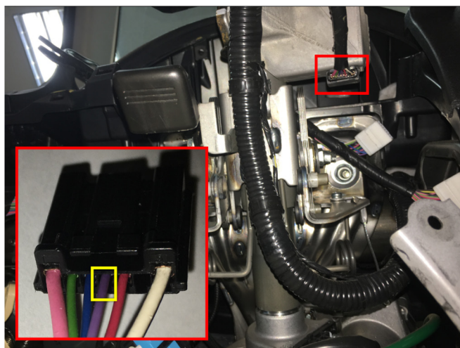
Разблокировка руля (фиолетовый провод)
