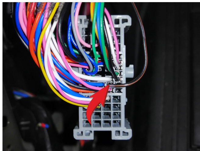
Шина данных (черный/оранжевый провод)
