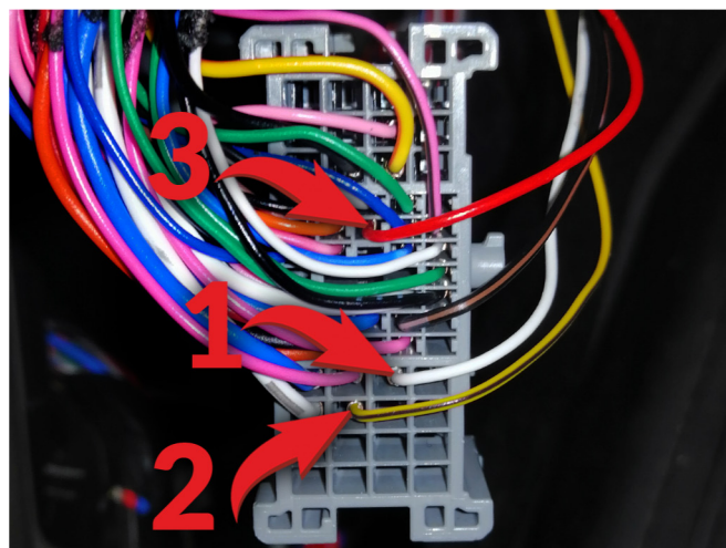
Подключение к цепям автозапуска 1 – Зажигание 1 (белый провод); 2 – Зажигание 2 (желтый/черный провод); 3 – Стартер (красный провод).
