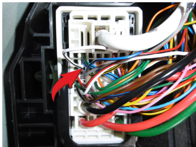
Шина данных (белый/черный провод)
