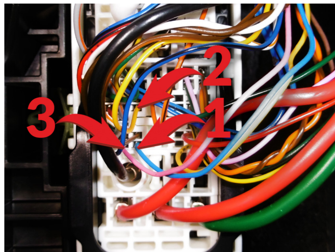
Подключение к цепям автозапуска 1 – Зажигание 1 (синий провод); 2 – Зажигание 2 (желтый провод); 3 – Стартер (розовый провод).
