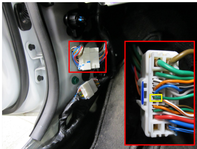
Шина данных (зеленый провод, контакт №19)
