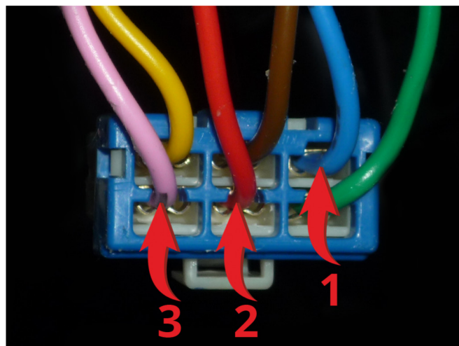
Подключение к силовым цепям запуска двигателя 1 - Зажигание 1 (синий провод); 2 - Зажигание 2 (красный провод); 3 - Стартер (розовый провод).
