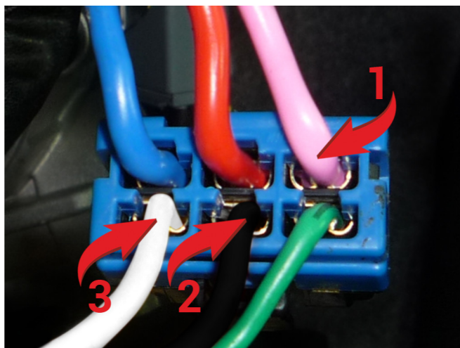
Подключение к силовым цепям запуска двигателя 1 – Зажигание 1 (розовый провод); 2 – Зажигание 2 (черный провод); 3 – Стартер (белый провод).
