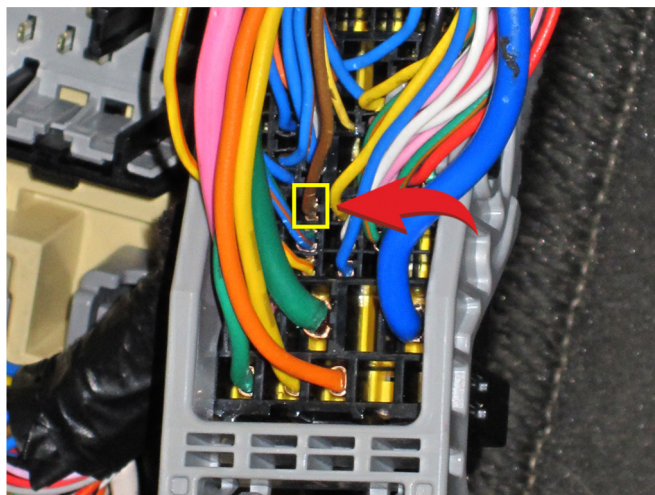
Шина данных (коричневый/оранжевый провод, контакт №55)
