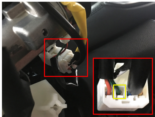
Ключ в замке (зеленый/черный провод)
