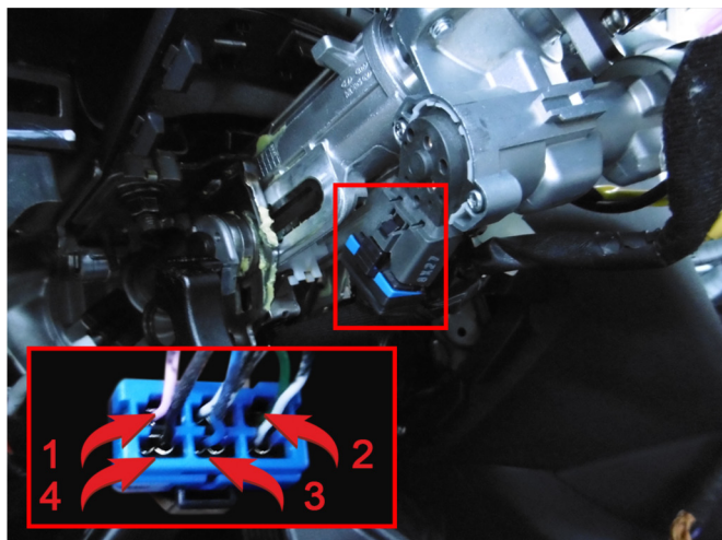
Подключение к силовым цепям запуска двигателя 1 – АСС (розовый провод); 2 – Зажигание 1 (зеленый провод); 3 – Зажигание 2 (синий провод); 4 – Стартер (чечный провод).
