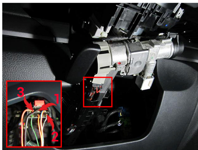
Подключение к цепям запуска двигателя 1 – Зажигание 1 (черный провод); 2 – Зажигание 2 (черный/белый провод); 3 – Стартер (оранжевый/черный провод).
