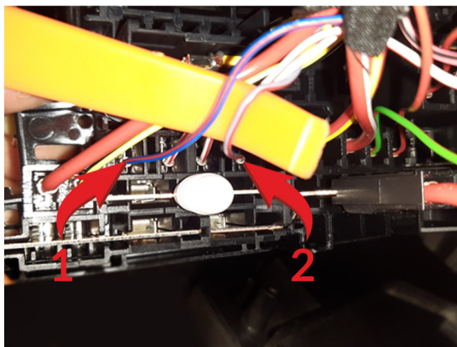
Подключение стартера: 1 – Стартер «-» (синий/красный провод); 2 – Стартер «-» (серый/красный провод)
