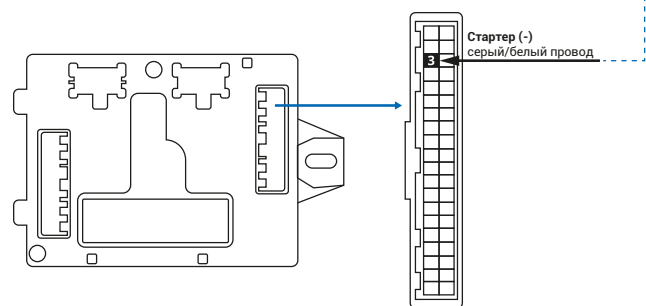
Рис.2 Схема подключения автозапуска
