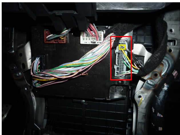
Рис.3 Место подключение стартера у блока BCM
