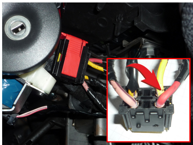
Рис.4 Место подключения силовых цепей у замка зажигания
