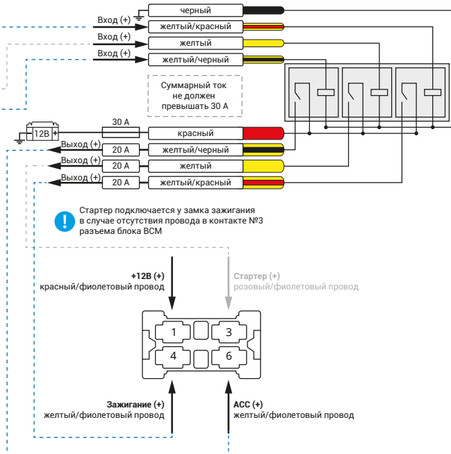
Рис.2 Схема подключения автозапуска
